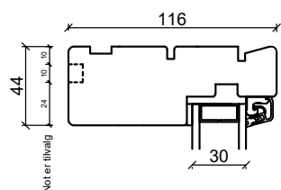
Overkarm
