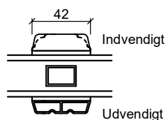
42 mm energisprosse
