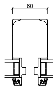
Lodpost
