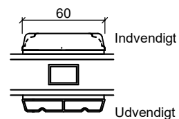
60 mm energisprosse
