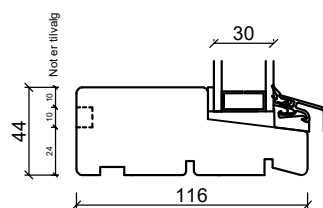
Bundkarm
