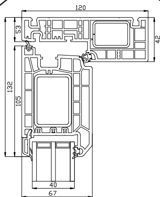
Overkarm
