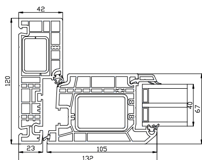
Sidekarm
