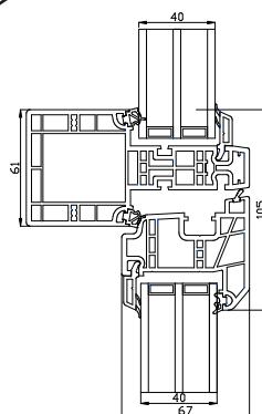
Tverrpost
