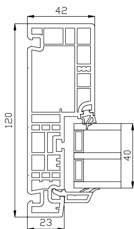
Sidekarm
