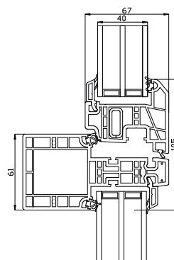
Tverrpost
