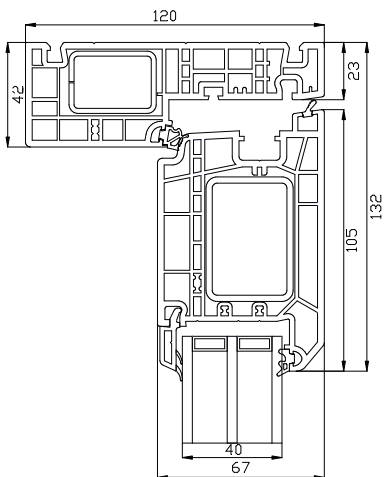
Overkarm
