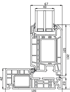
Bunnkarm
