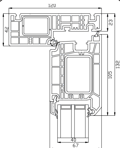
Overkarm
