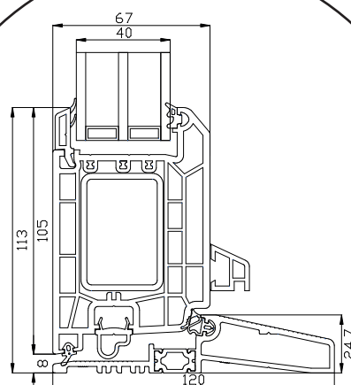
Bunnkarm
